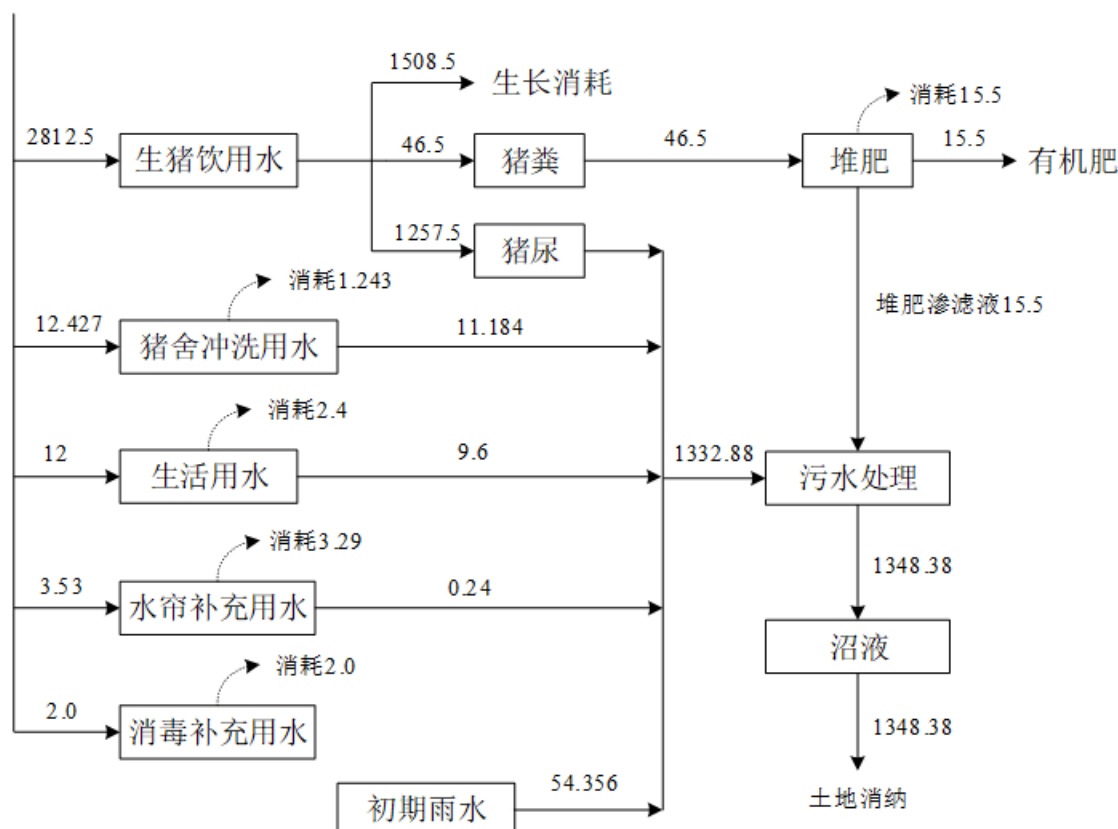
图 3.3.3-1 本项目夏季水平衡图 单位：t/d
