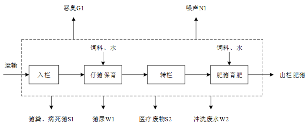
图 3.3.2-1 营运期工艺流程及产污节点图
