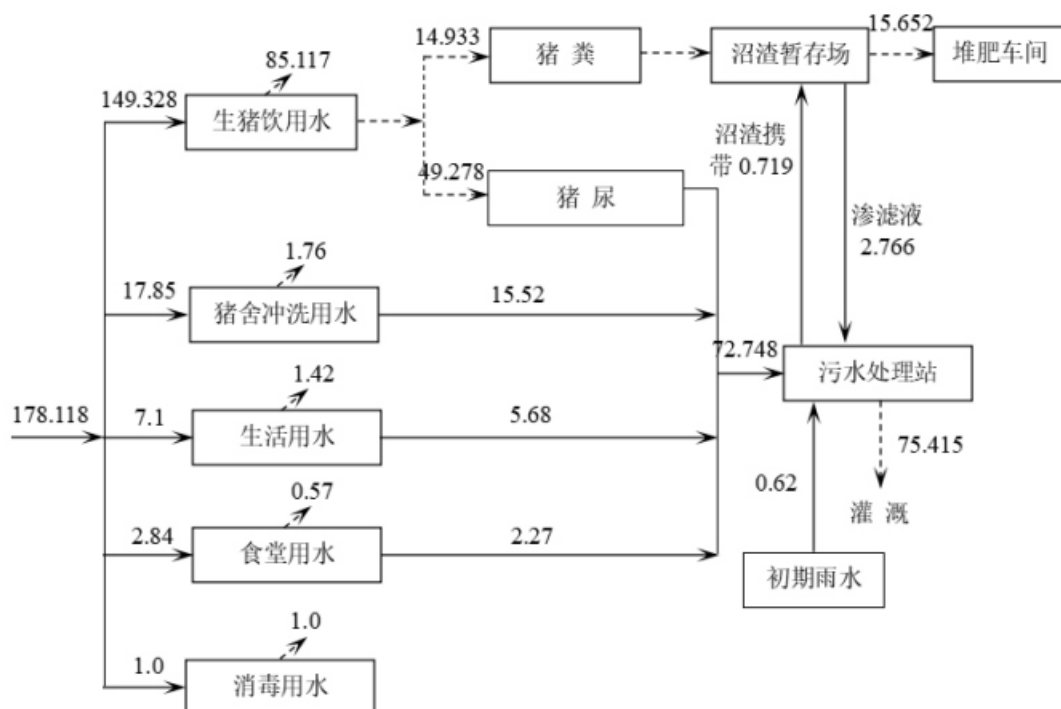
图 2.1.8-2 其他季水平衡图 (单位: \text{m}^3/\text{d} )
