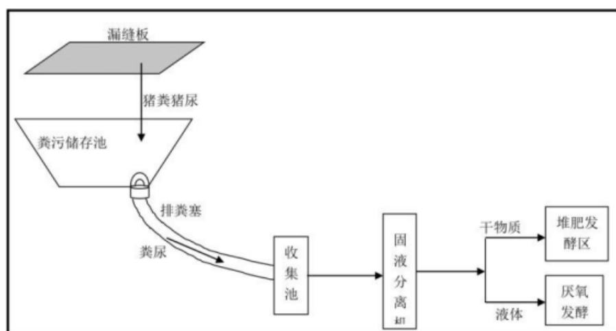
图 3.3.2-3 项目清粪工艺示意图
