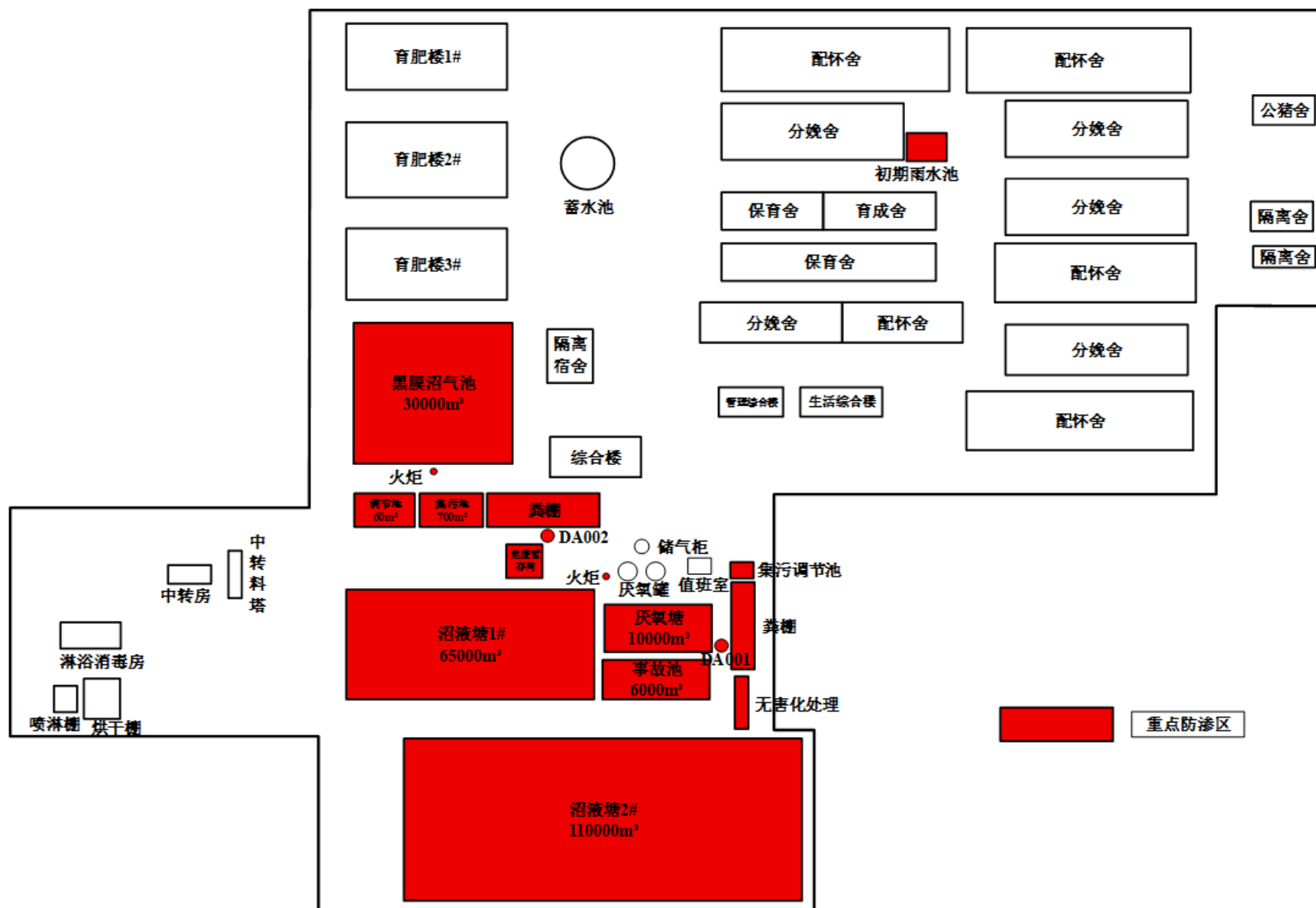
图 7.2.5-1 项目分区防渗图
