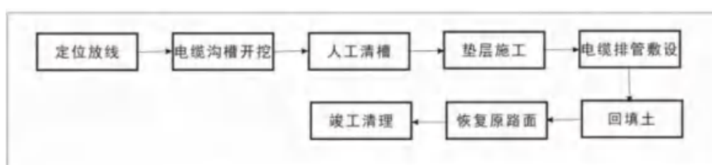
图 2.3-1 敞开式开挖施工工艺流程图
