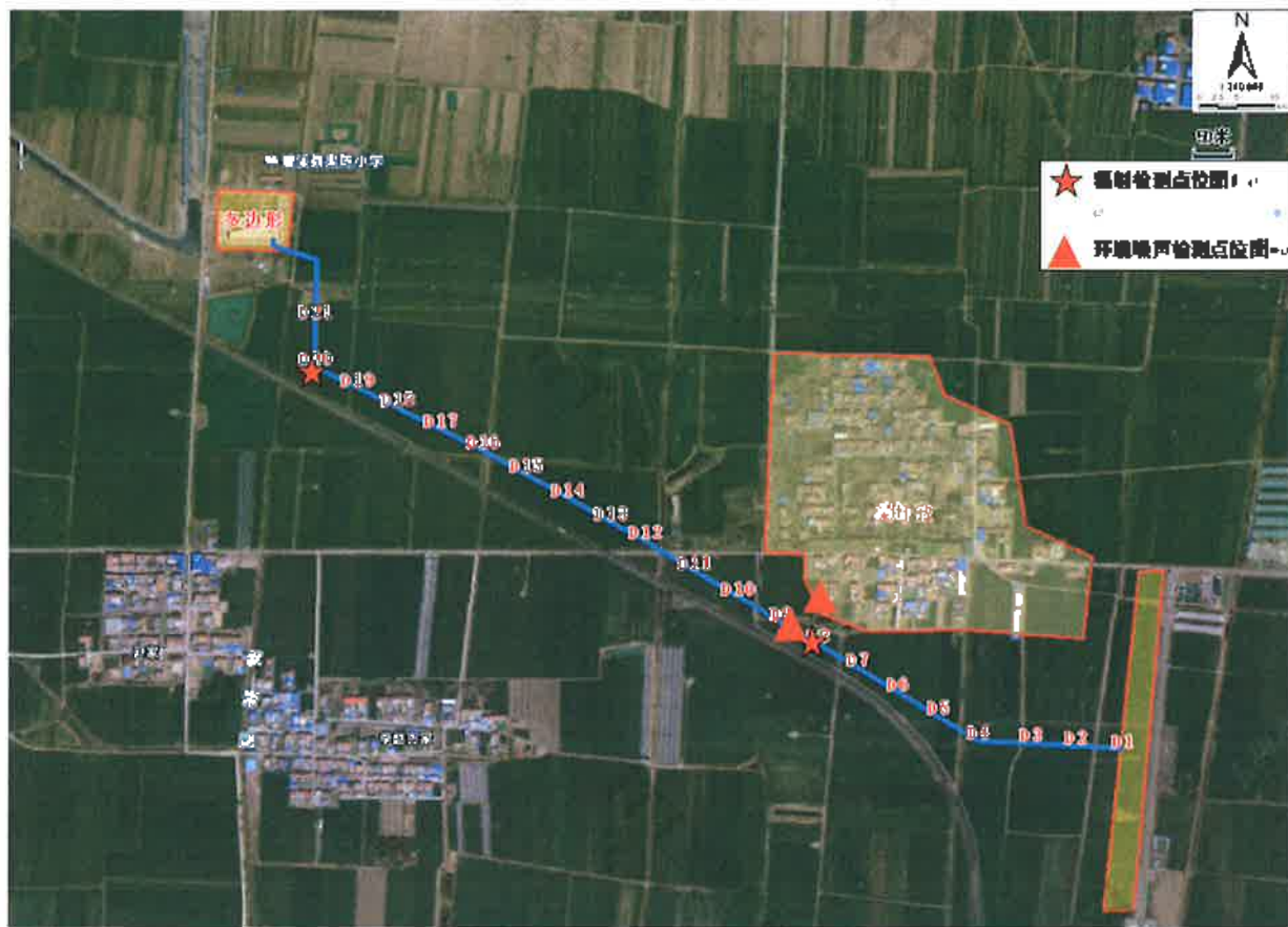
图 6-1 辐射、环境噪声检测点位示意图
