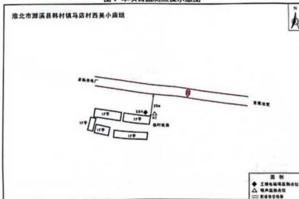
图 2 本项目监测点位示意图
