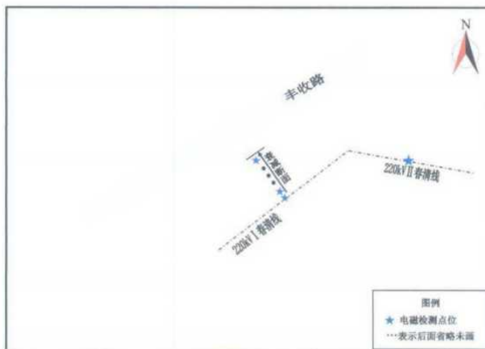
图 3 220kV 春清线单回电缆线路检测布点图
