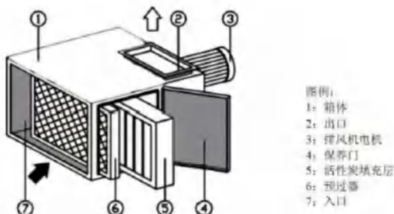
图 7.1-2 活性炭吸附工作原理图
