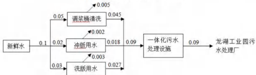
图 3.2-6 一期水平衡图 单位: t/d
