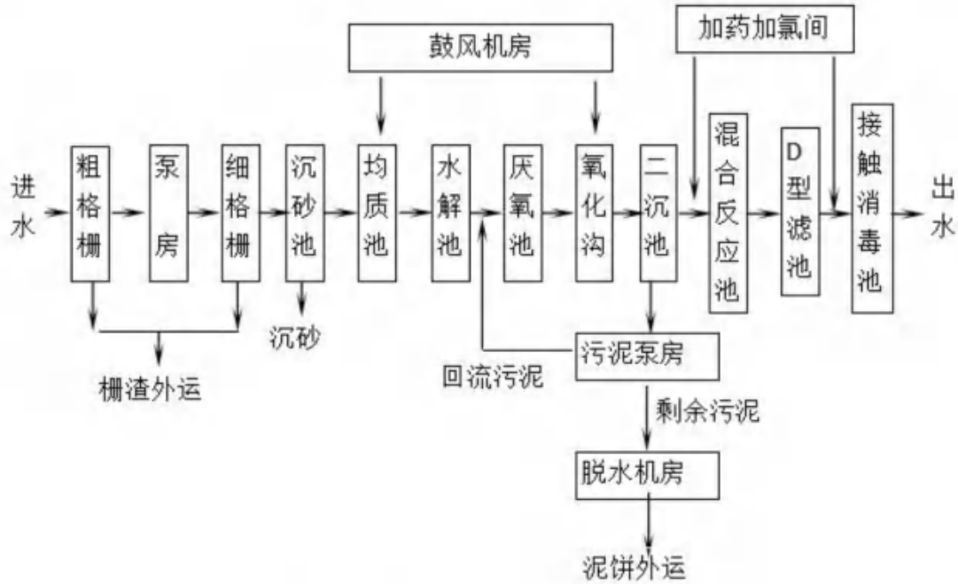
图 5.2-8 龙湖污水处理厂工艺流程图
