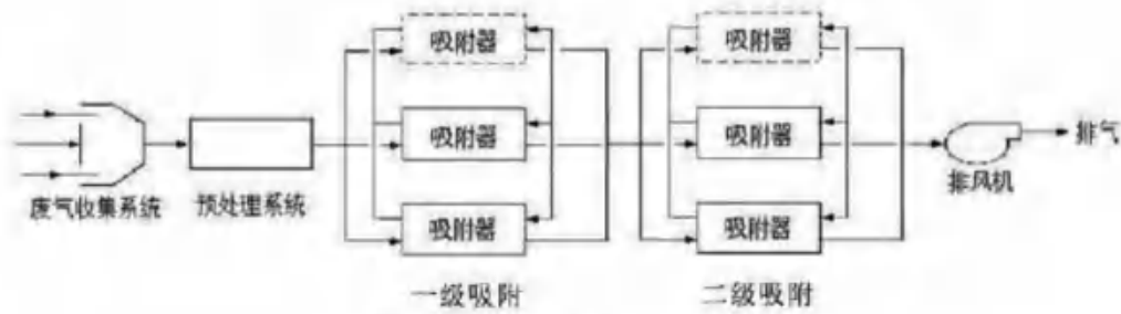
图 7.1-3 活性炭处置装置示意图
