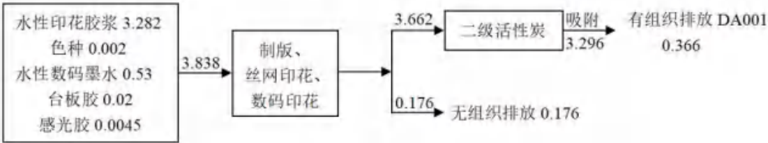
图 3.2-4 一期工程非甲烷总烃平衡图 (t/a)
