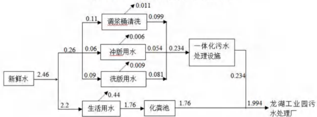
图 3.2-7 二期水平衡图 单位: t/d
