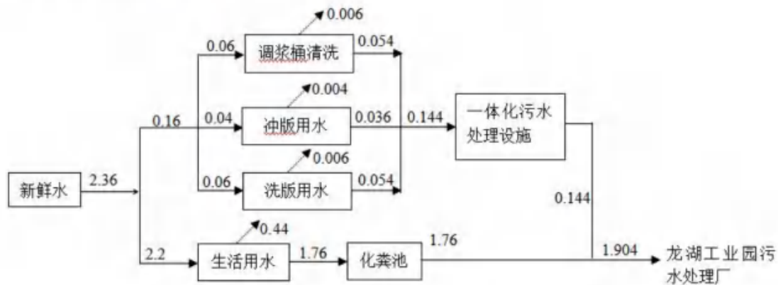
图 3.2-6 一期水平衡图 单位: t/d
