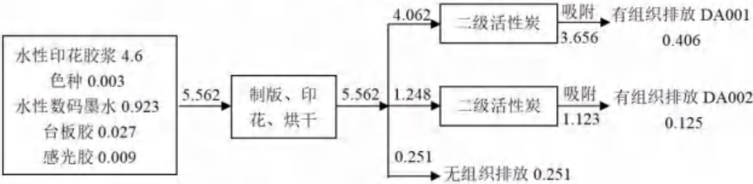
图 3.2-5 二期后全厂非甲烷总烃平衡图 (t/a)
