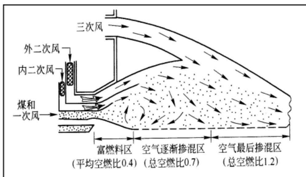
图 6.2.2-1 空气分级燃烧原理示意图
