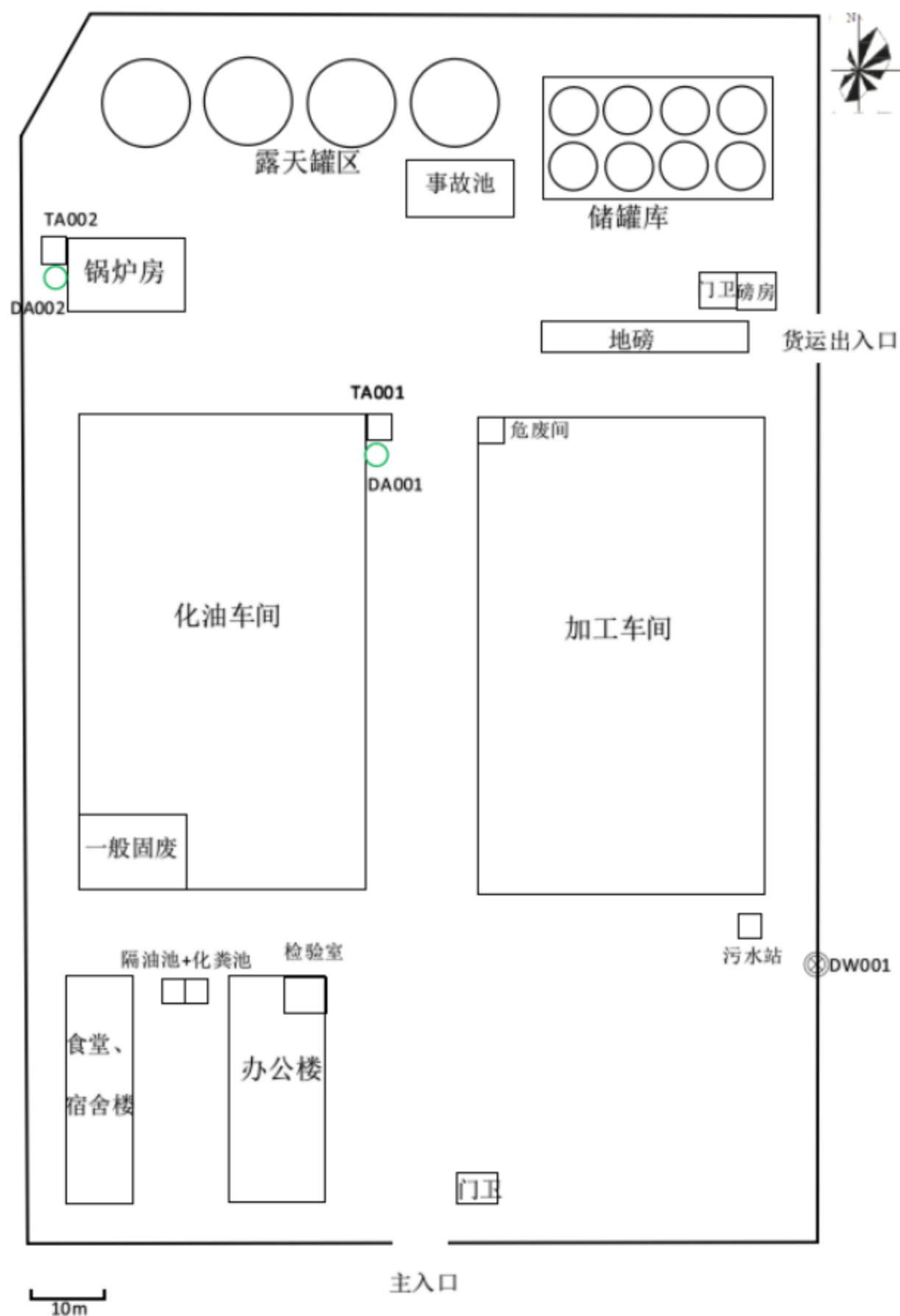
图3.2-2 厂区总平面布置图
