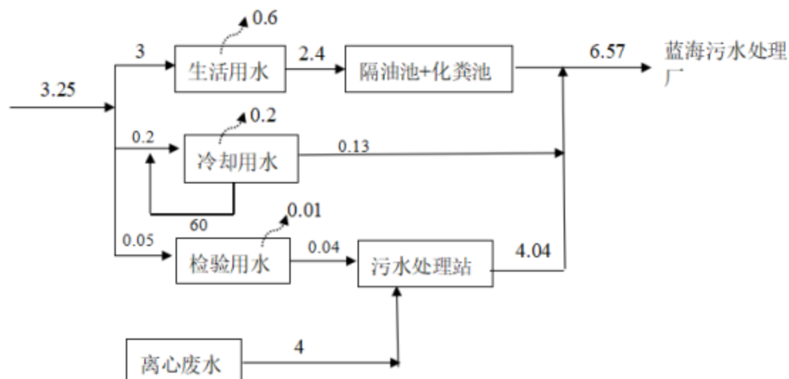
图3.3-3 本项目水平衡图 \text{m}^3/\text{d}
