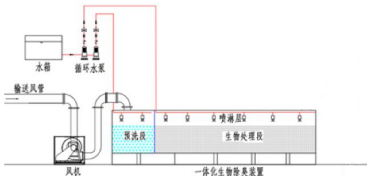
图 3.3-1 除臭工艺流程示意图
