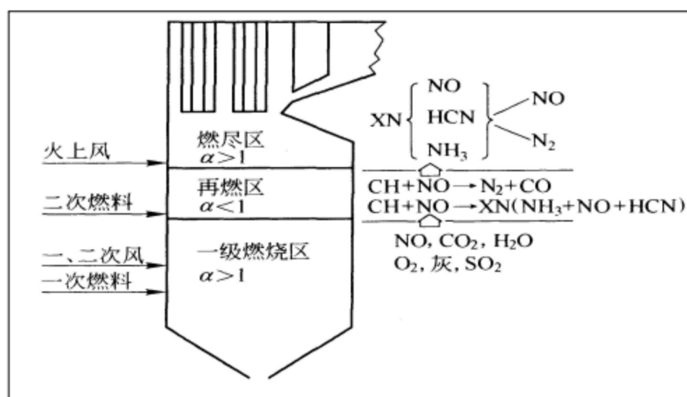
图 6.2.2-2 燃料分级燃烧原理示意图
