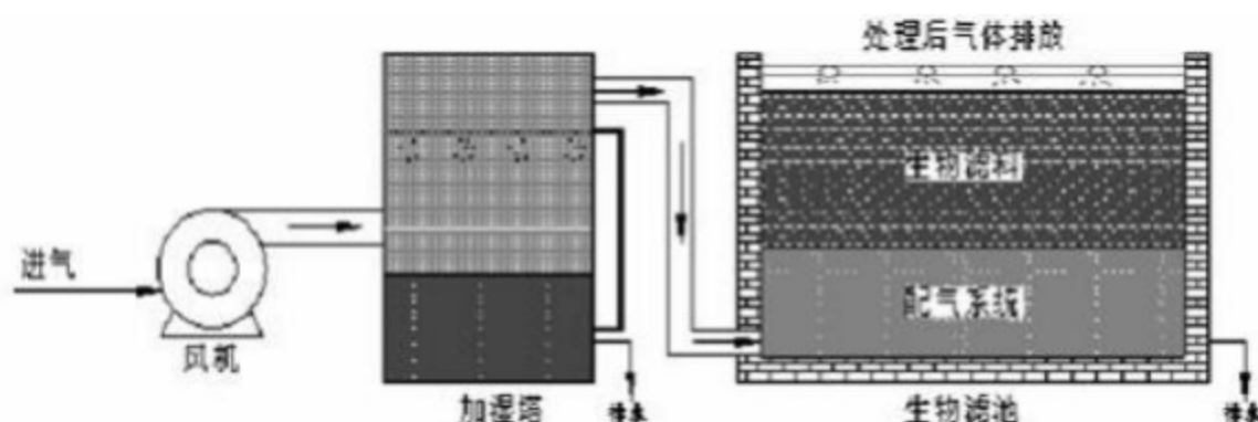
图 6.2.1-1 生物除臭系统示意图
