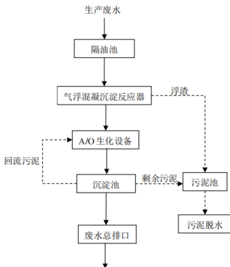
图 6.1.2-1 污水处理站工艺流程图
