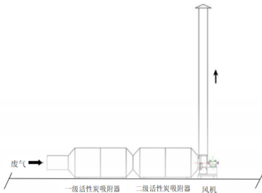
图 6.2.1-2 “二级活性炭吸附装置”工艺流程图
