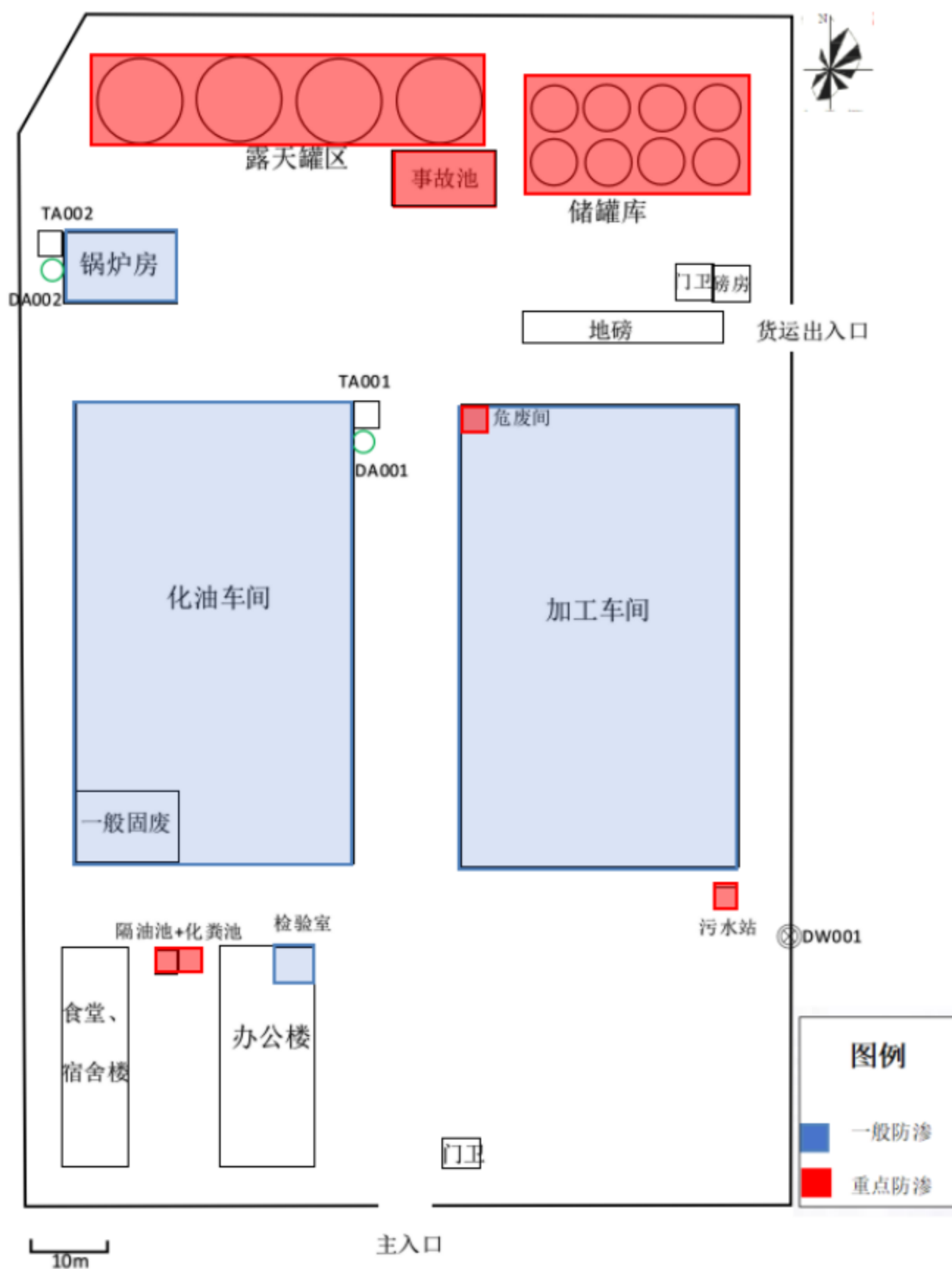
图 6.5-1 分区防渗图
