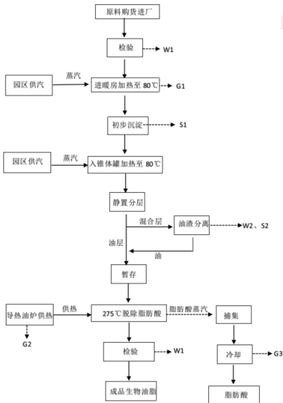
图 3.3-1 工艺流程及产污节点图
