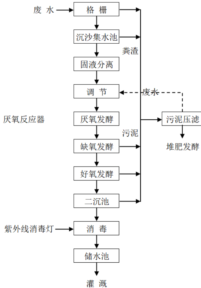
图 6.2-3 项目粪污处理工艺流程图
