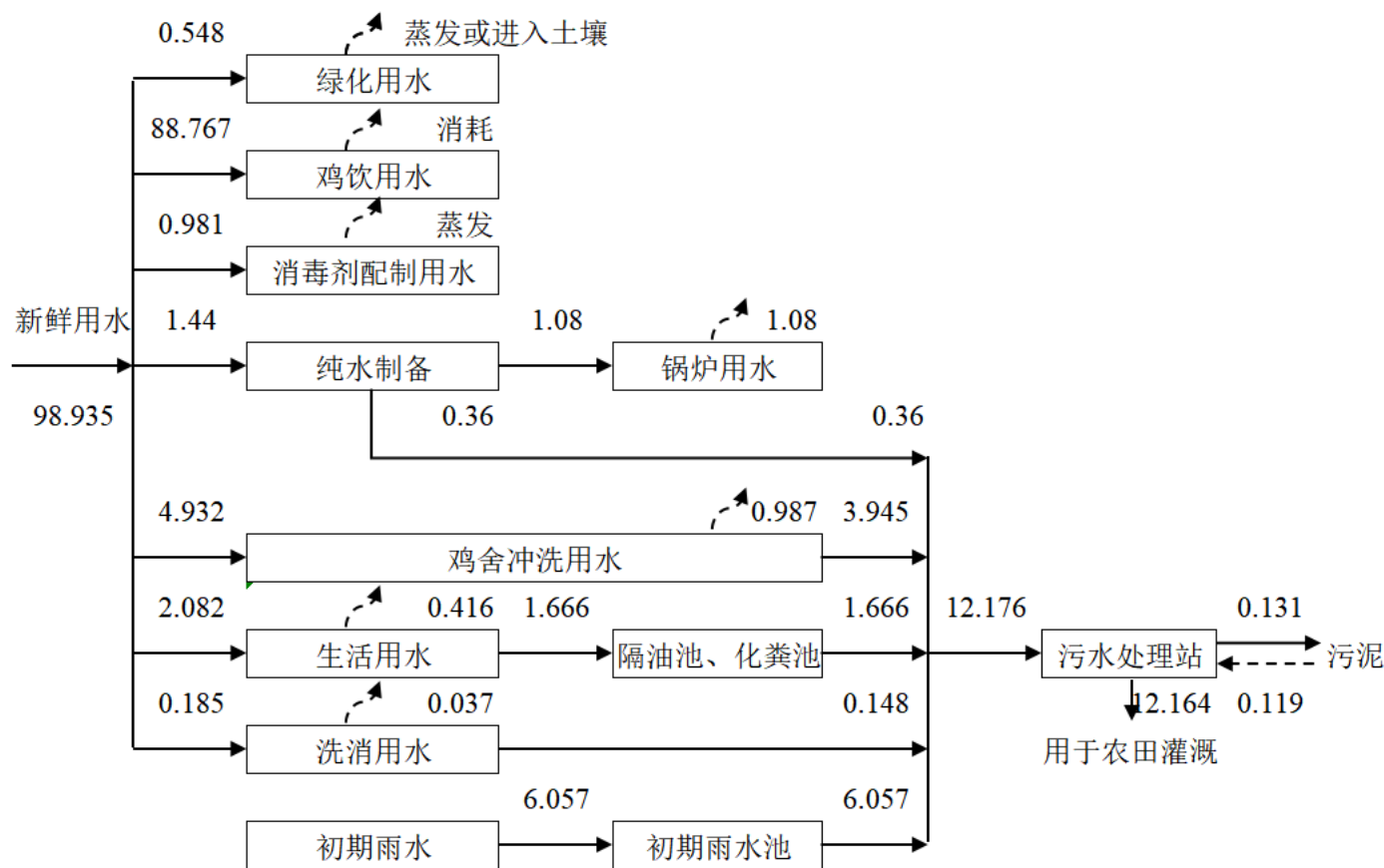
图 3.5-3 本项目其它季节水平衡图 (单位: m³/d, 200d)
