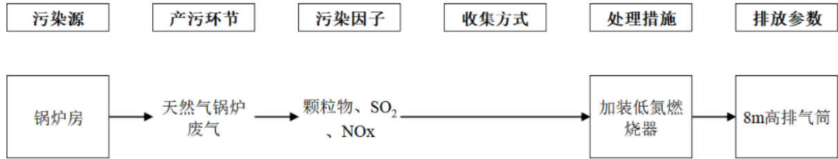
图 6.2-1 本项目废气收集处理管线图
