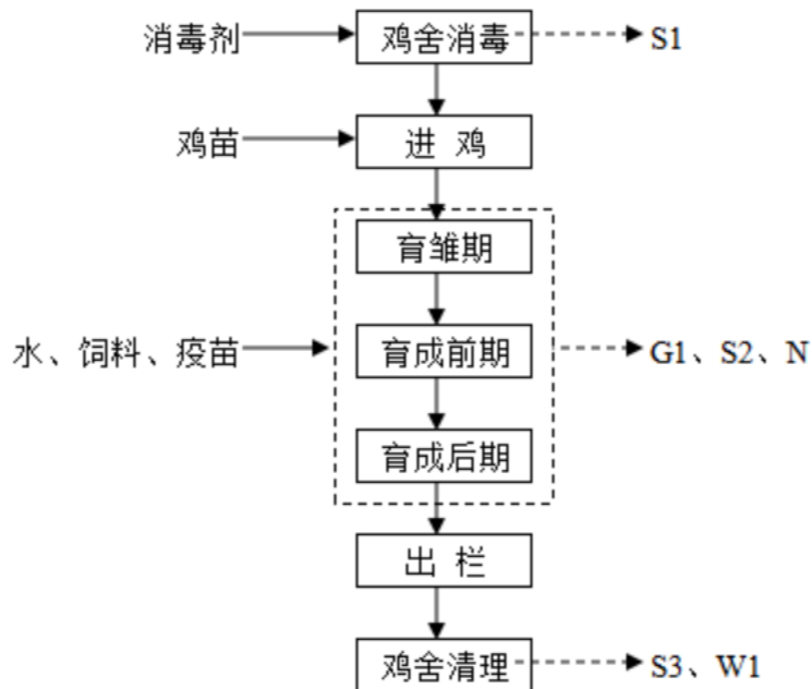
图 3.4-1 养殖工艺流程和产污节点图
