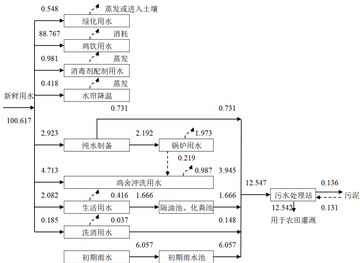
图 3.5-1 本项目水平衡图 (单位: m³/d, 365d)
