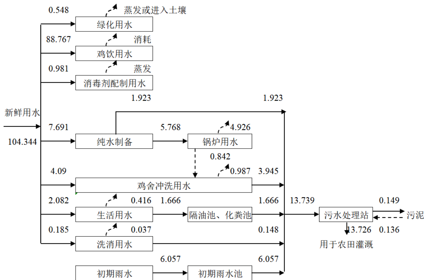
图 3.5-4 本项目冬季水平衡图 (单位: m 3 /d, 95d)
