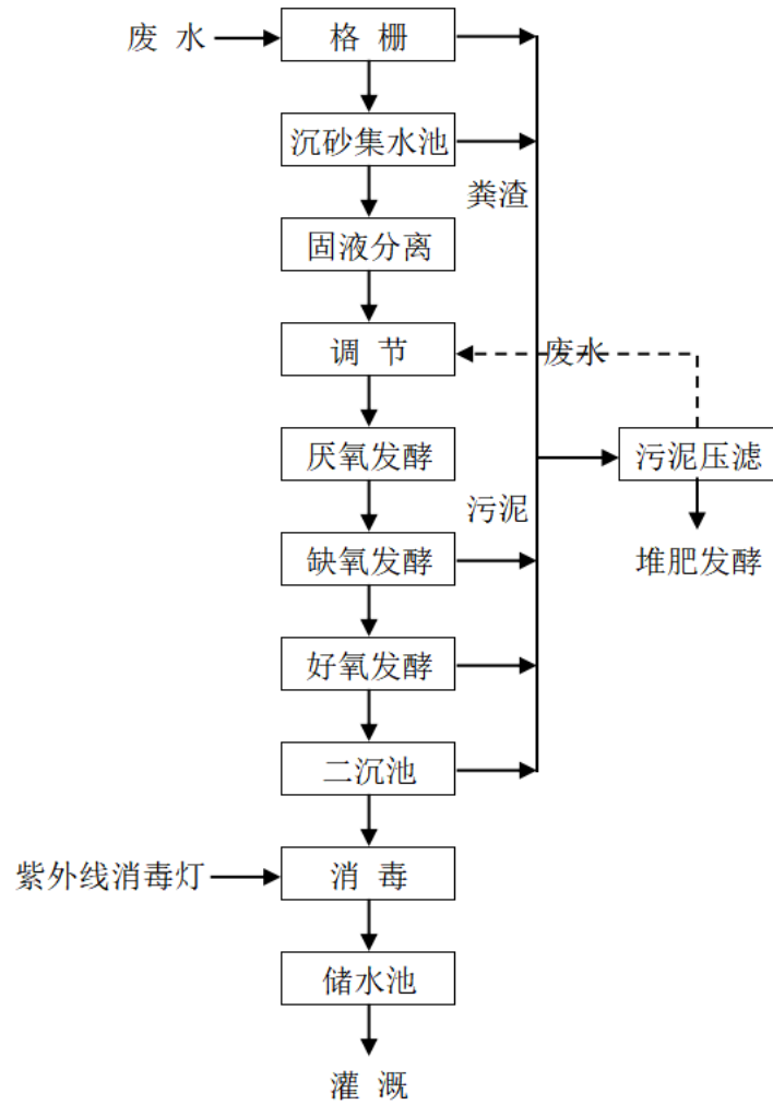
图 3.4-4 项目污水处理工艺流程图
