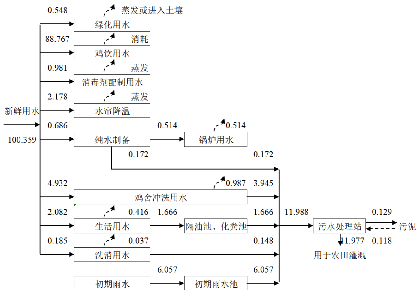
图 3.5-2 本项目夏季水平衡图 (单位: m 3 /d, 70d)
