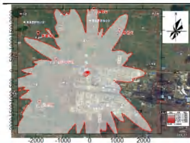
图 5.2.5-1 SO 2 小时平均贡献浓度分布图 µg/m 3
