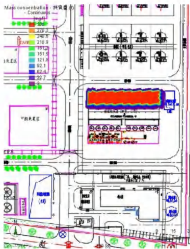
图 5.6.6-1 非正常工况下 100d 后耗氧量迁移平面图
