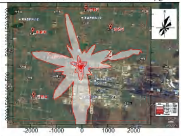
图 5.2.5-16 非甲烷总烃小时平均浓度图 \mu\text{g}/\text{m}^3
