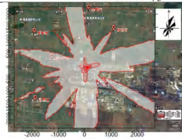
图 5.2.5-12 硫化氢小时平均贡献浓度图 \mu\text{g}/\text{m}^3
