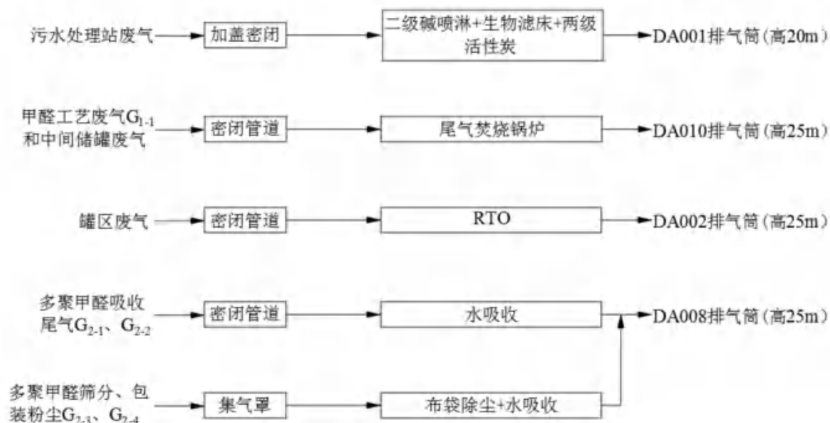
图 6.1.1-1 重新报批后项目废气收集处理工艺示意图
