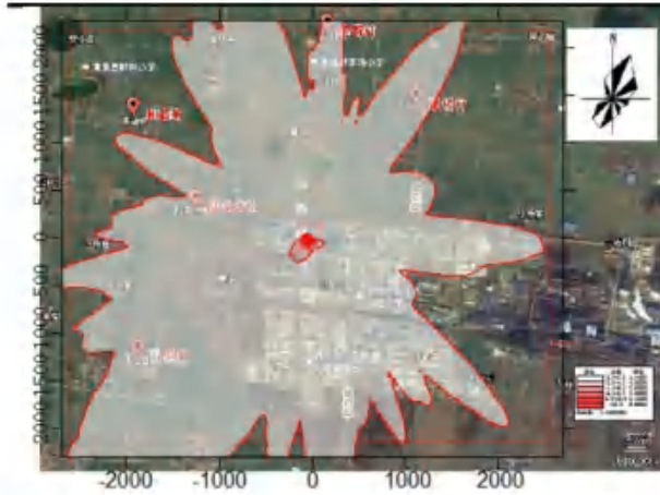
图 5.2.5-13 甲醛小时平均贡献浓度分布图 \mu\text{g}/\text{m}^3
