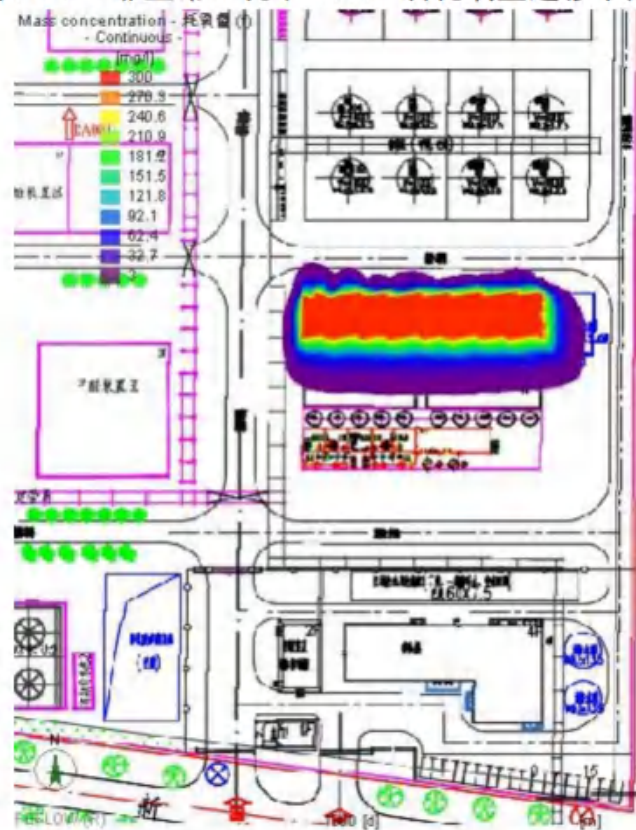
图 5.6.6-2 非正常工况下 1000d 后耗氧量迁移平面图
