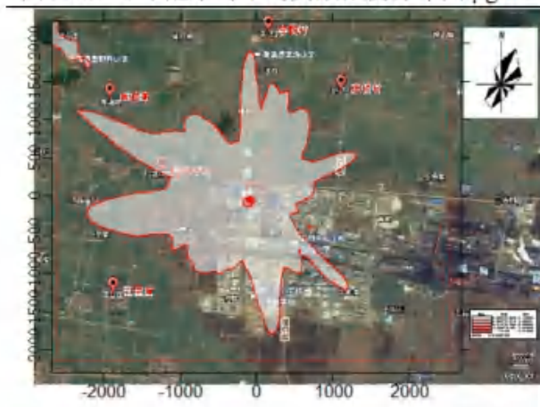
图 5.2.5-15 甲醇日平均贡献浓度分布图 \mu\text{g}/\text{m}^3
