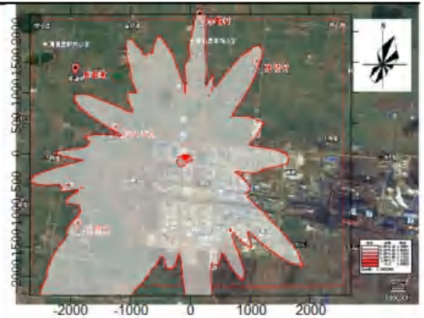
图 5.2.5-14 甲醇小时平均贡献浓度分布图 \mu\text{g}/\text{m}^3
