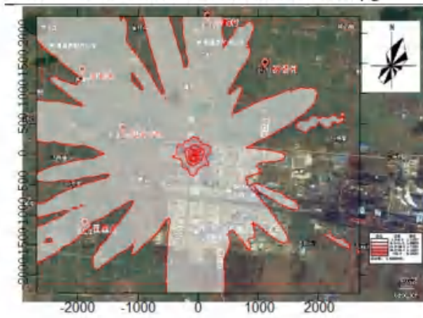
图 5.2.5-17 TSP 日平均贡献浓度分布图 \mu\text{g}/\text{m}^3
