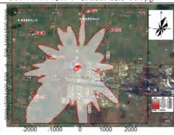
图 5.2.5-4 NO 2 小时平均贡献浓度分布图 µg/m 3
