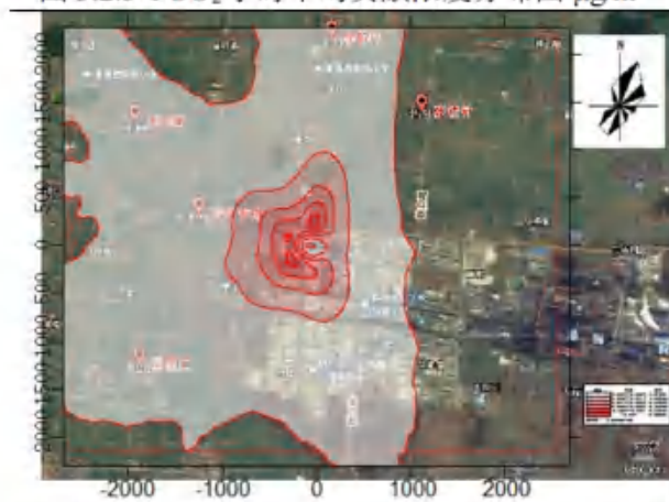
图 5.2.5-3 SO 2 年均贡献值浓度分布图 µg/m 3
