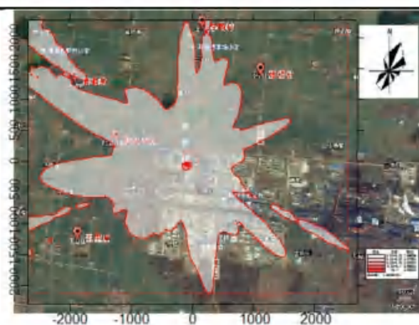
图 5.2.5-2 SO 2 日平均贡献浓度分布图 µg/m 3
