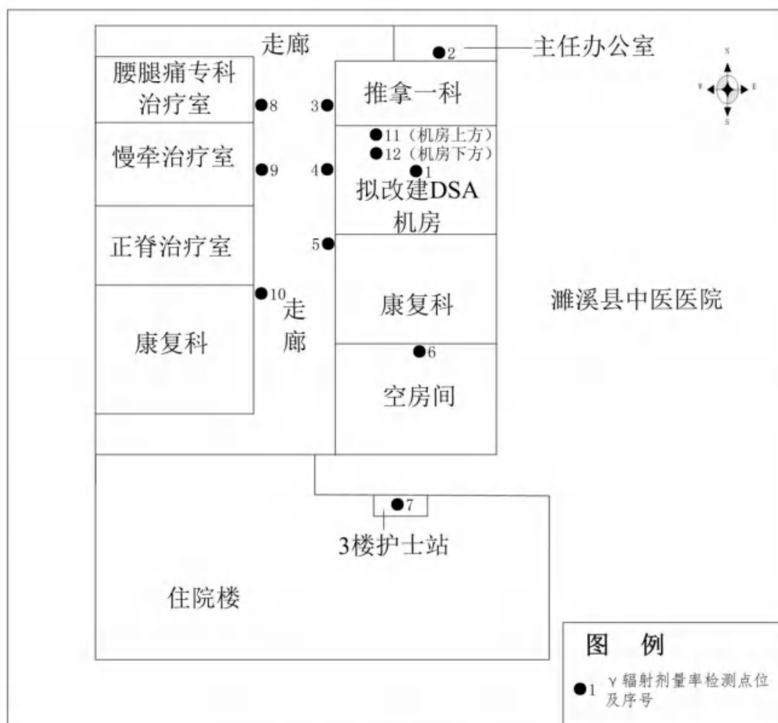
图 8-2 \gamma 辐射空气吸收剂量率测布点图
