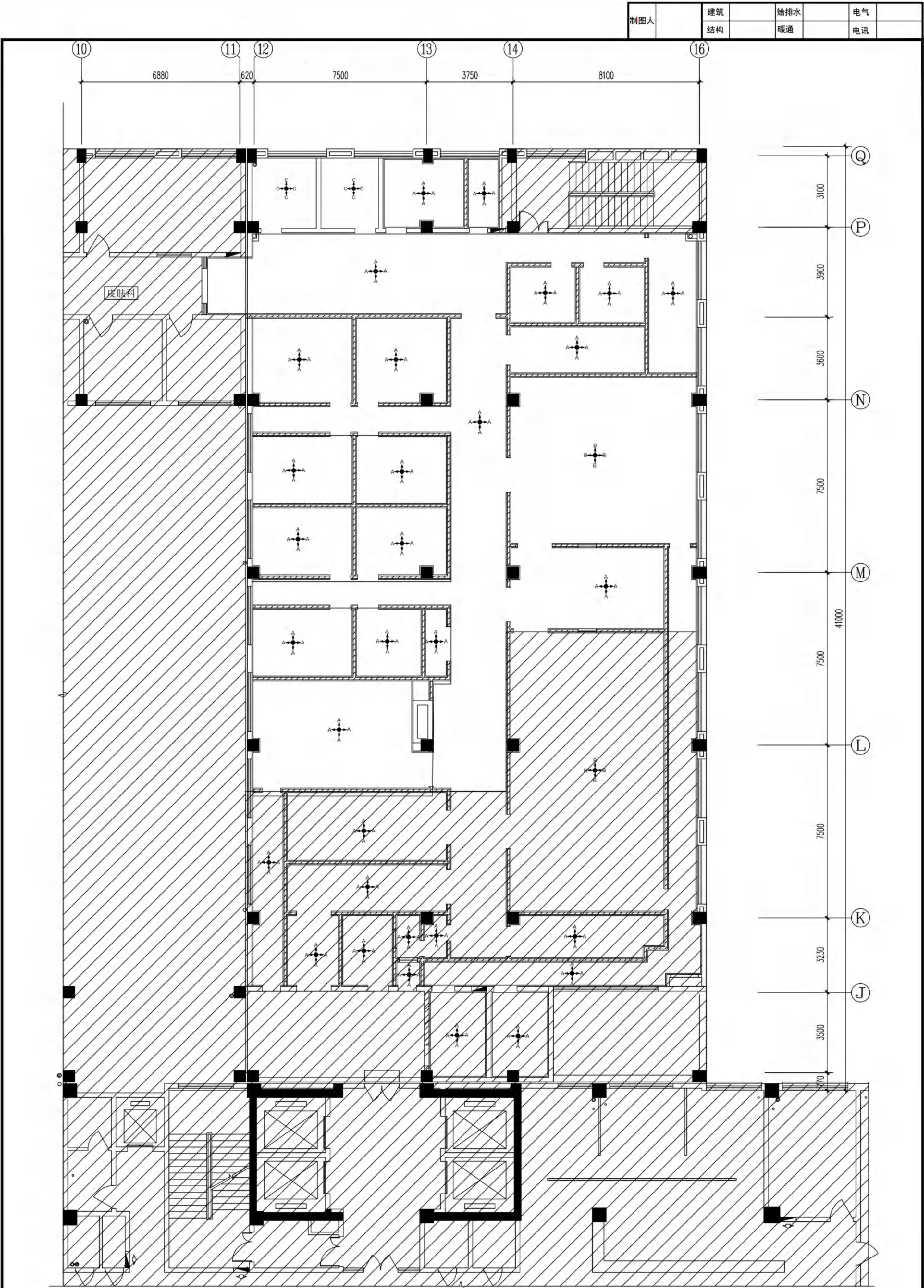
附图7 DSA机房新建墙体防护图 三层墙体材料图 1:100
