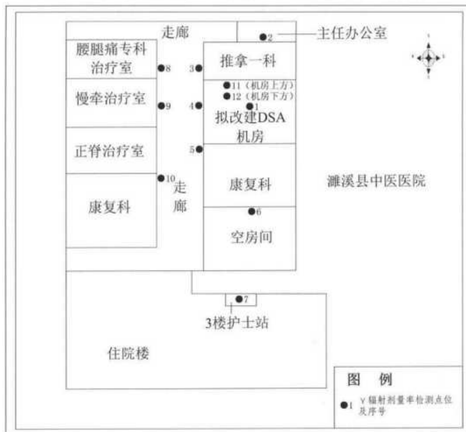
附图 1: 濉溪县中医医院拟改建 DSA 机房周围 \gamma 辐射剂量率检测布点示意图
