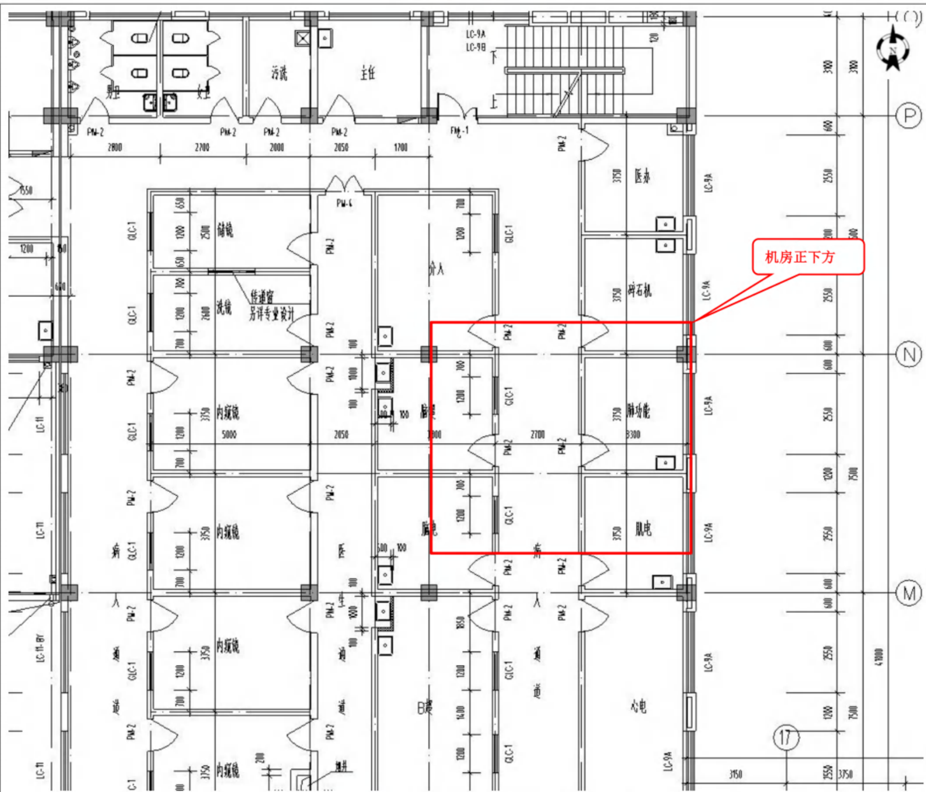
图 1-6 DSA 机房正下方（二层）平面布置图
