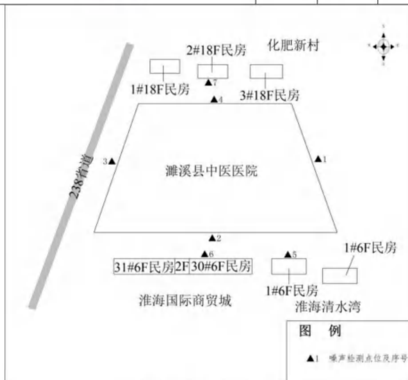
图 8-3 声环境监测布点图
