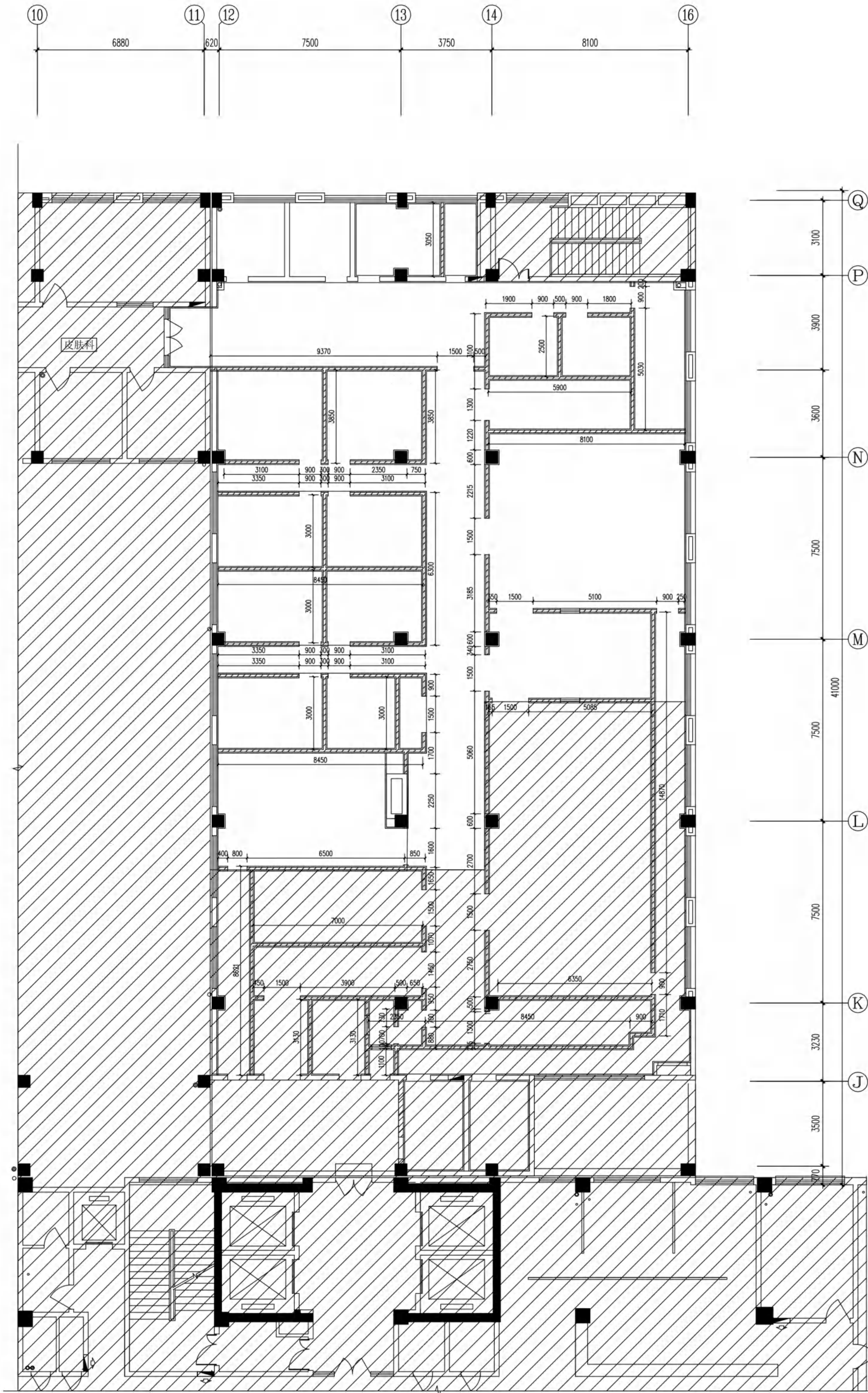
三层新建墙体尺寸图 1:100
