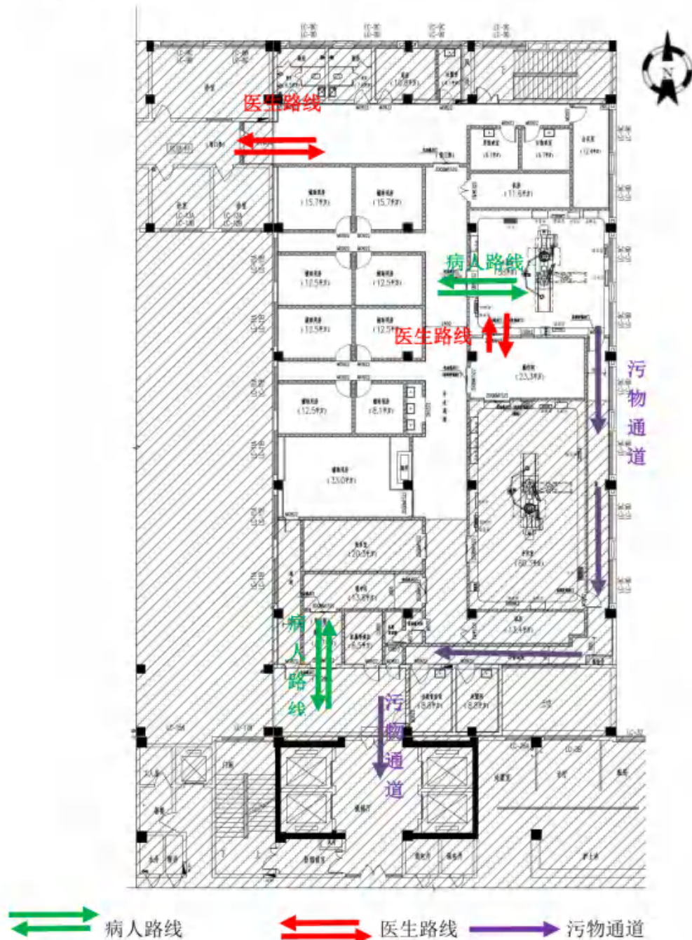
图 9-3 人流、物流路径规划图
