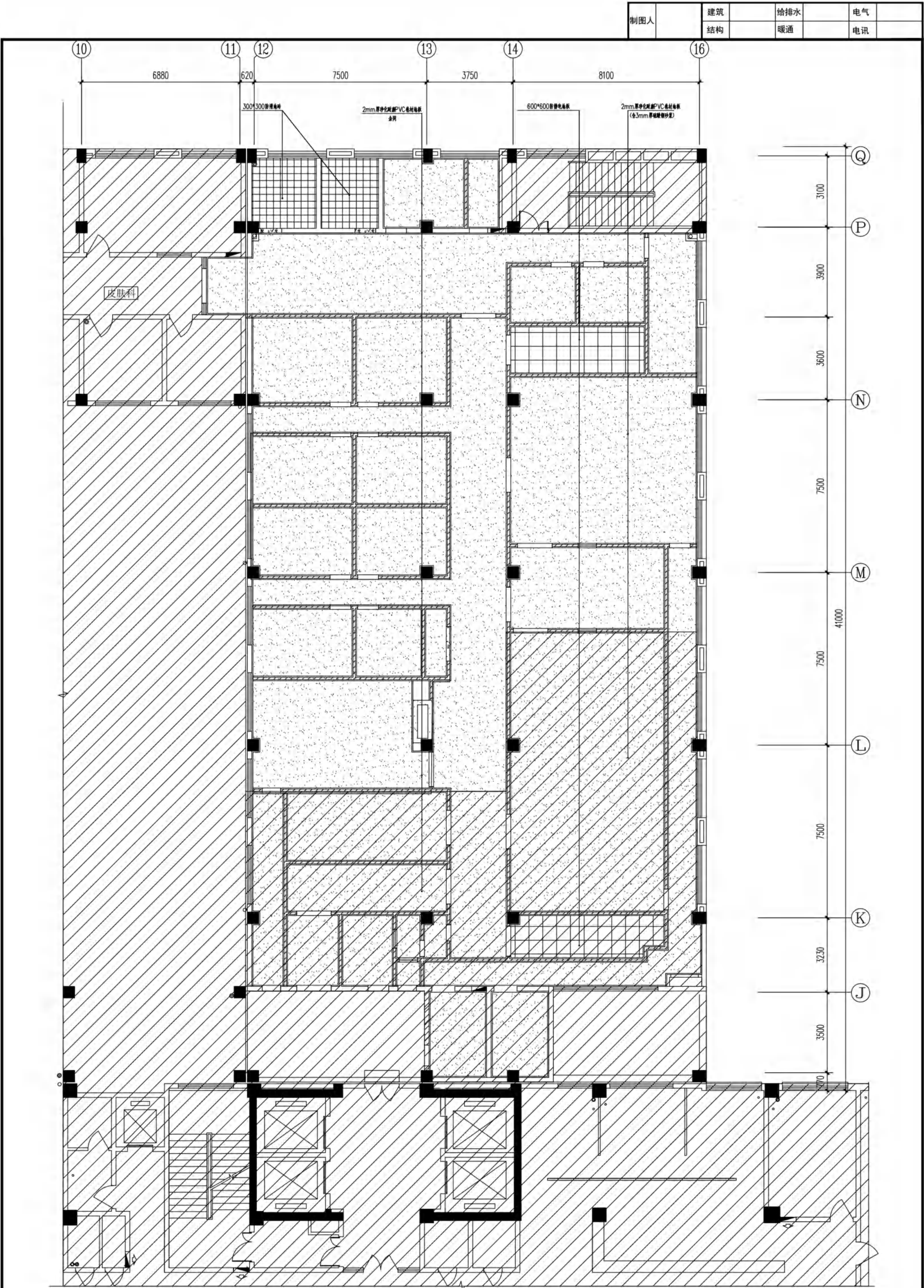
附图5 DSA机房地面防护图 三层地面布置图 1:100 注：三层楼板为100mm厚钢筋混凝土楼板。
