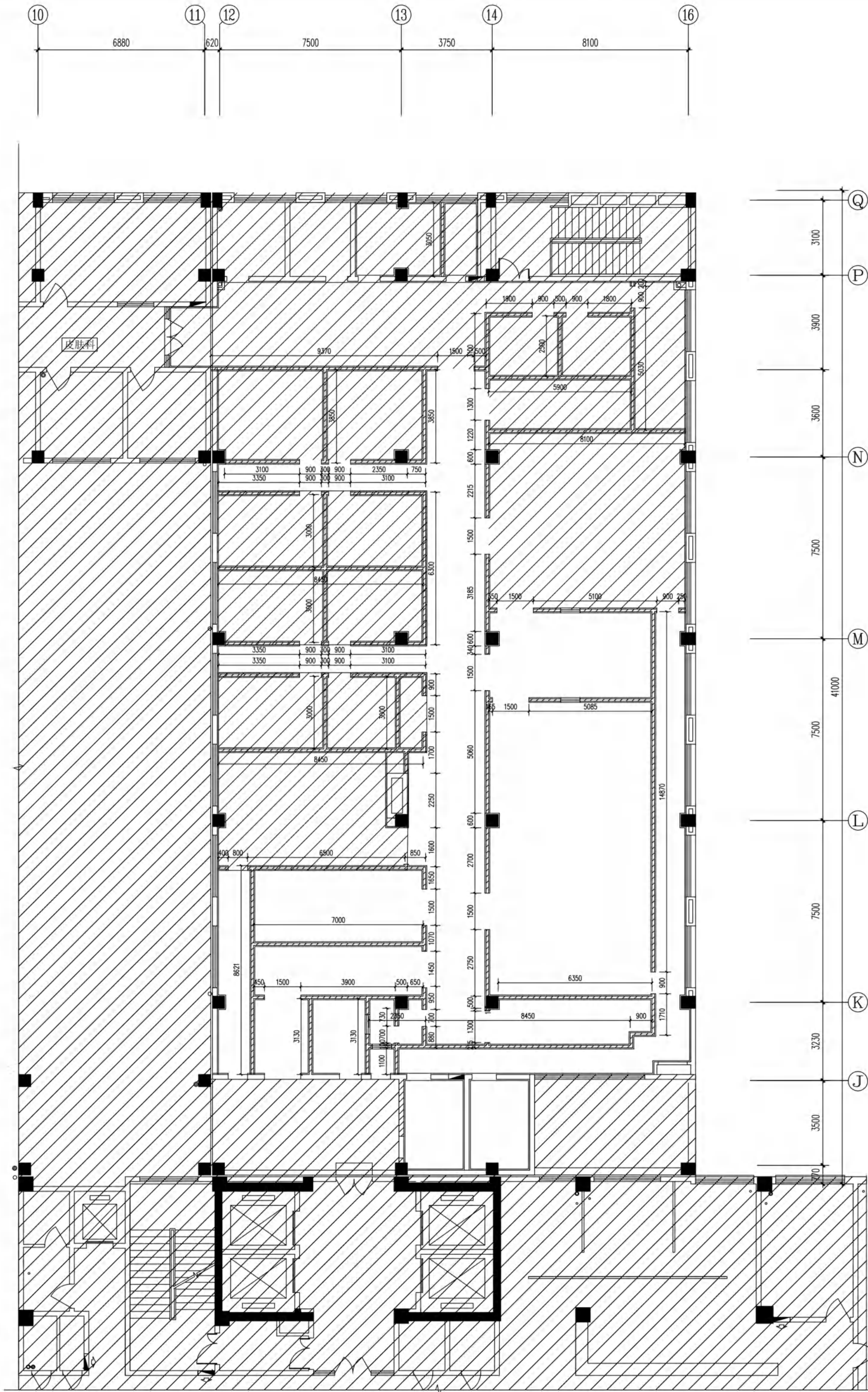
附图4 三层新建墙体尺寸图 1:100
