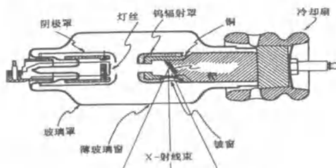
图 9-1 典型 X 射线管示意图
