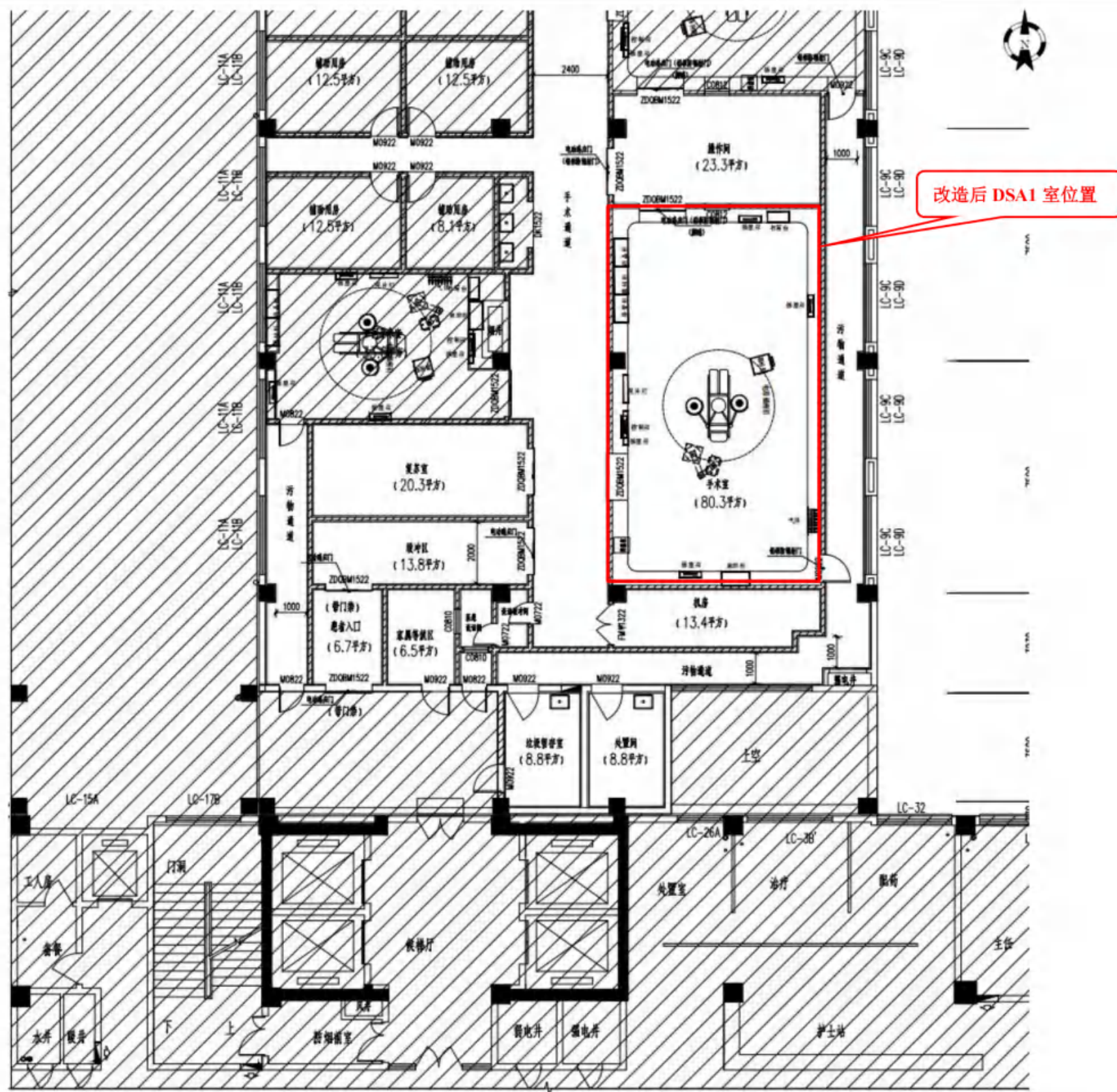
图 1-5 DSA 机房改建后所在三楼平面布置图
