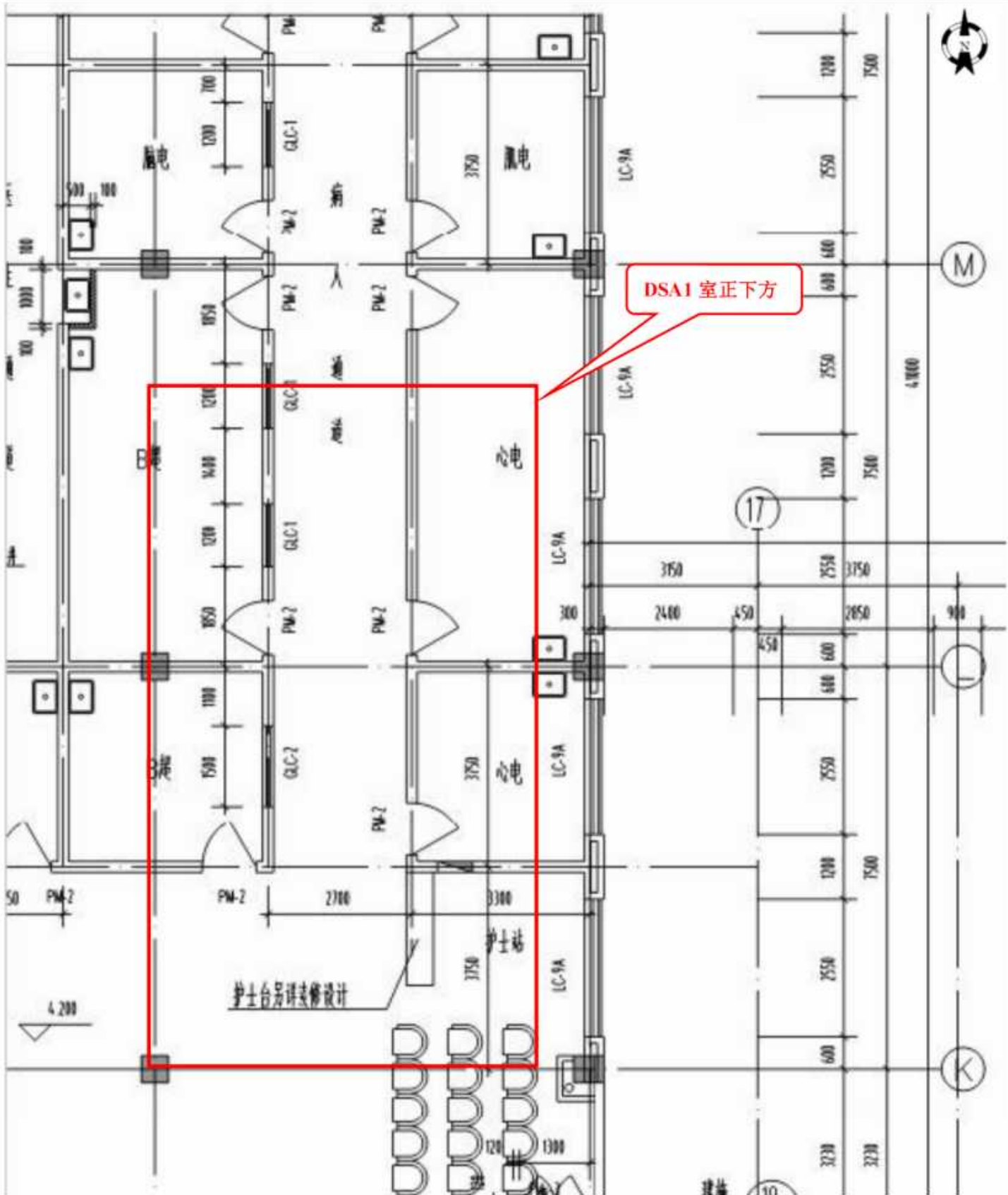
图 1-6 DSA 机房正下方（二层）平面布置图
