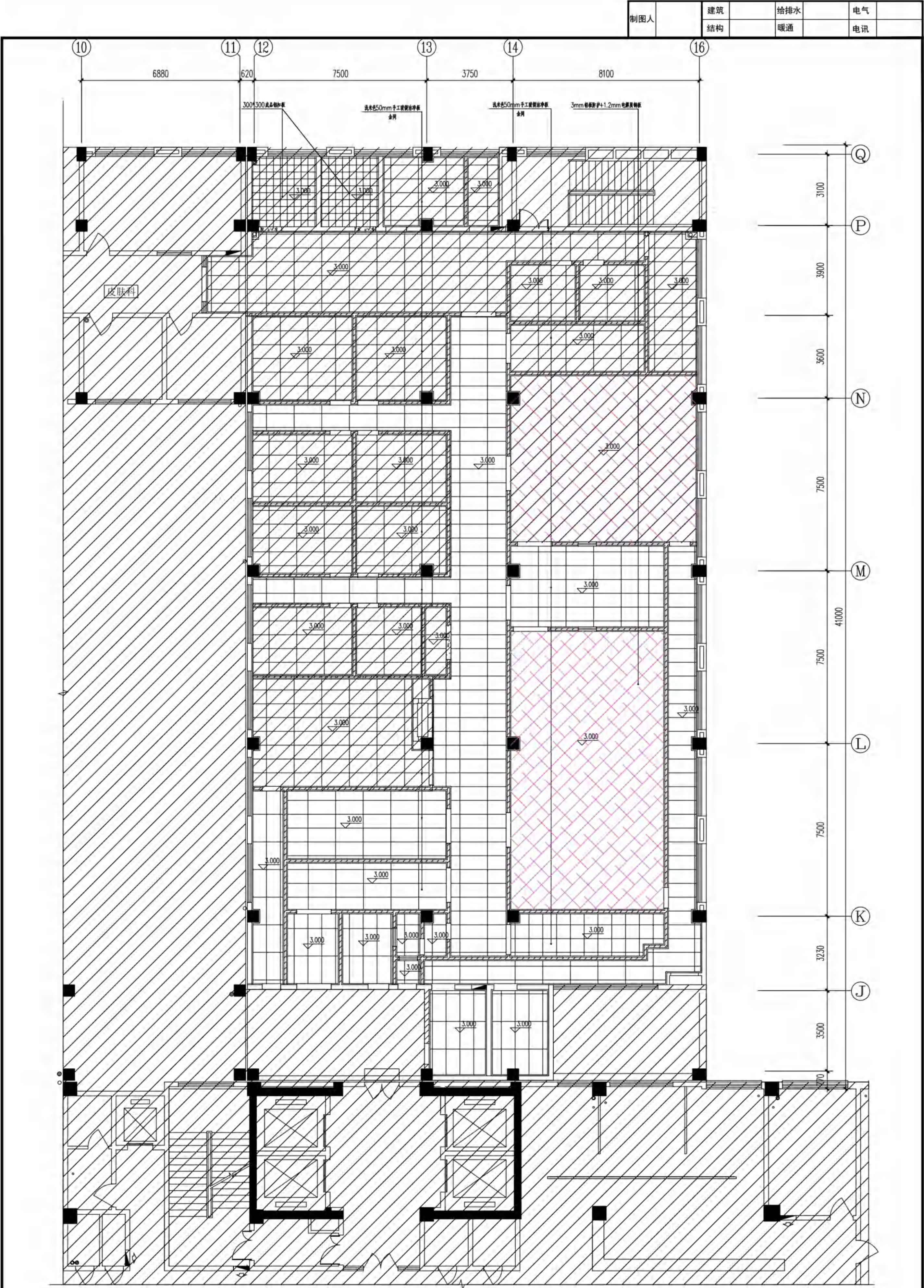
附图6 三层顶面布置图 1:100 注：四层楼板为100mm厚钢筋混凝土楼板。
