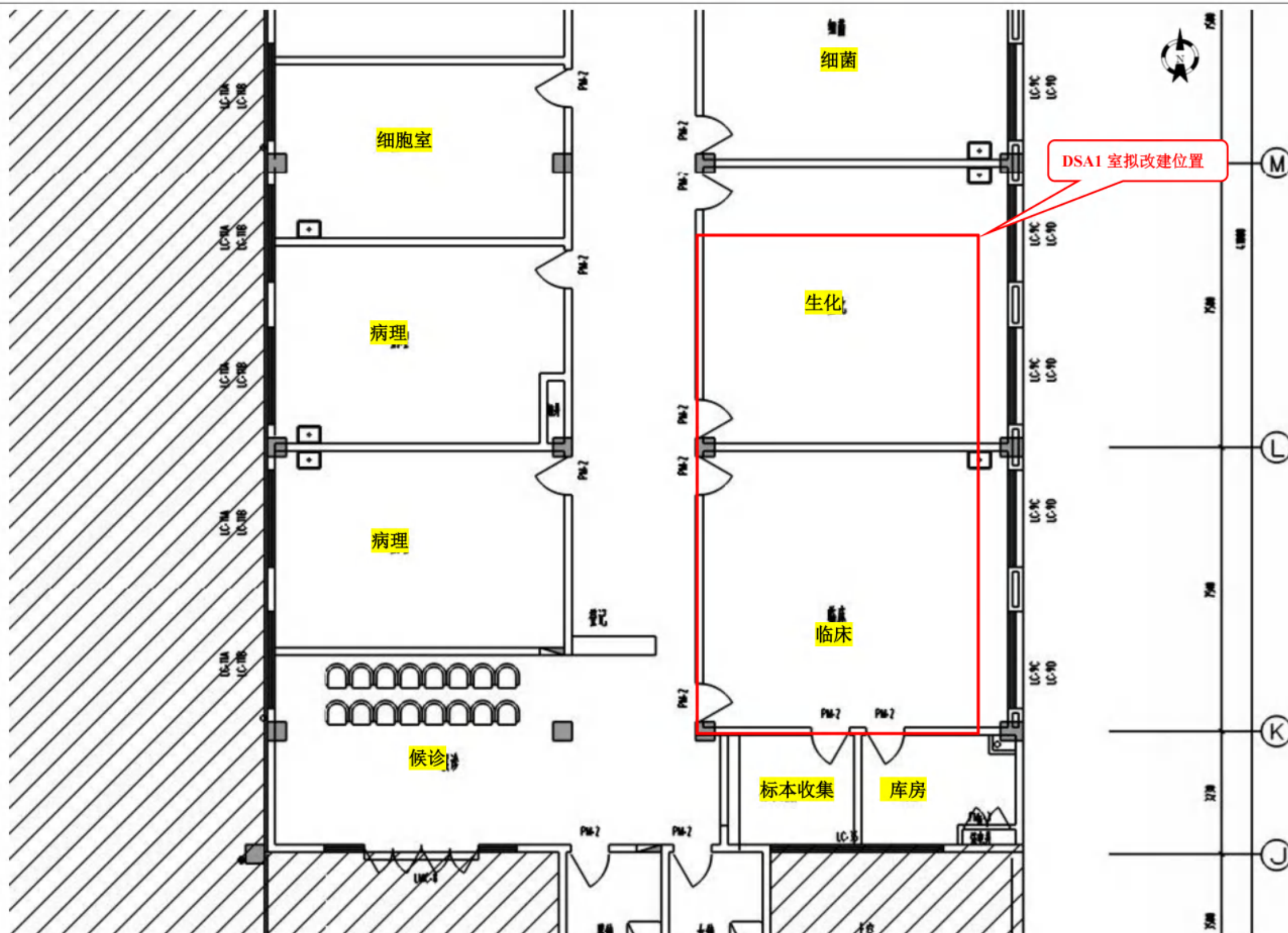
图 1-4 DSA 机房改建前所在三楼平面布置图
