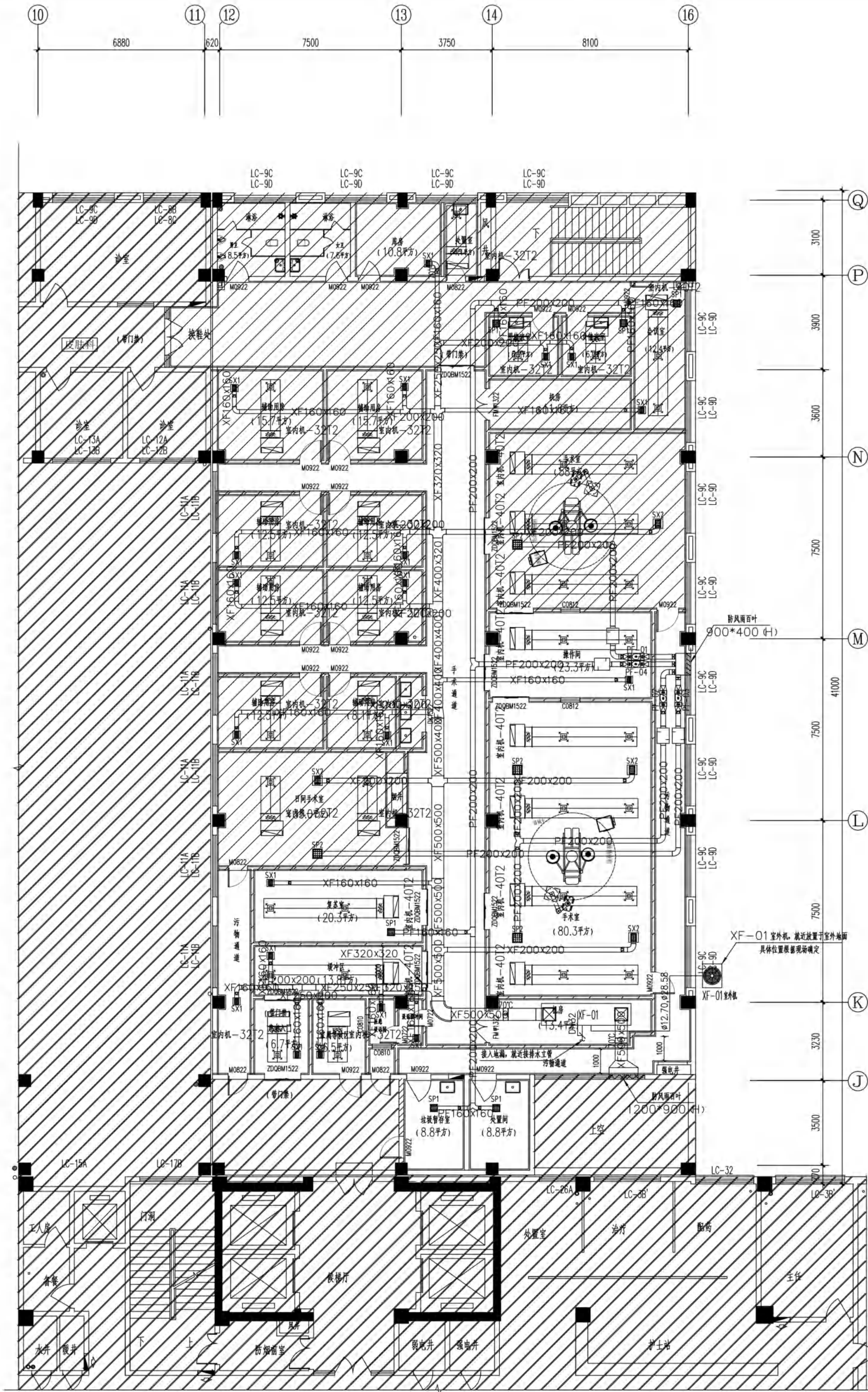
附图8 三层改造空调新风平面图1:100
