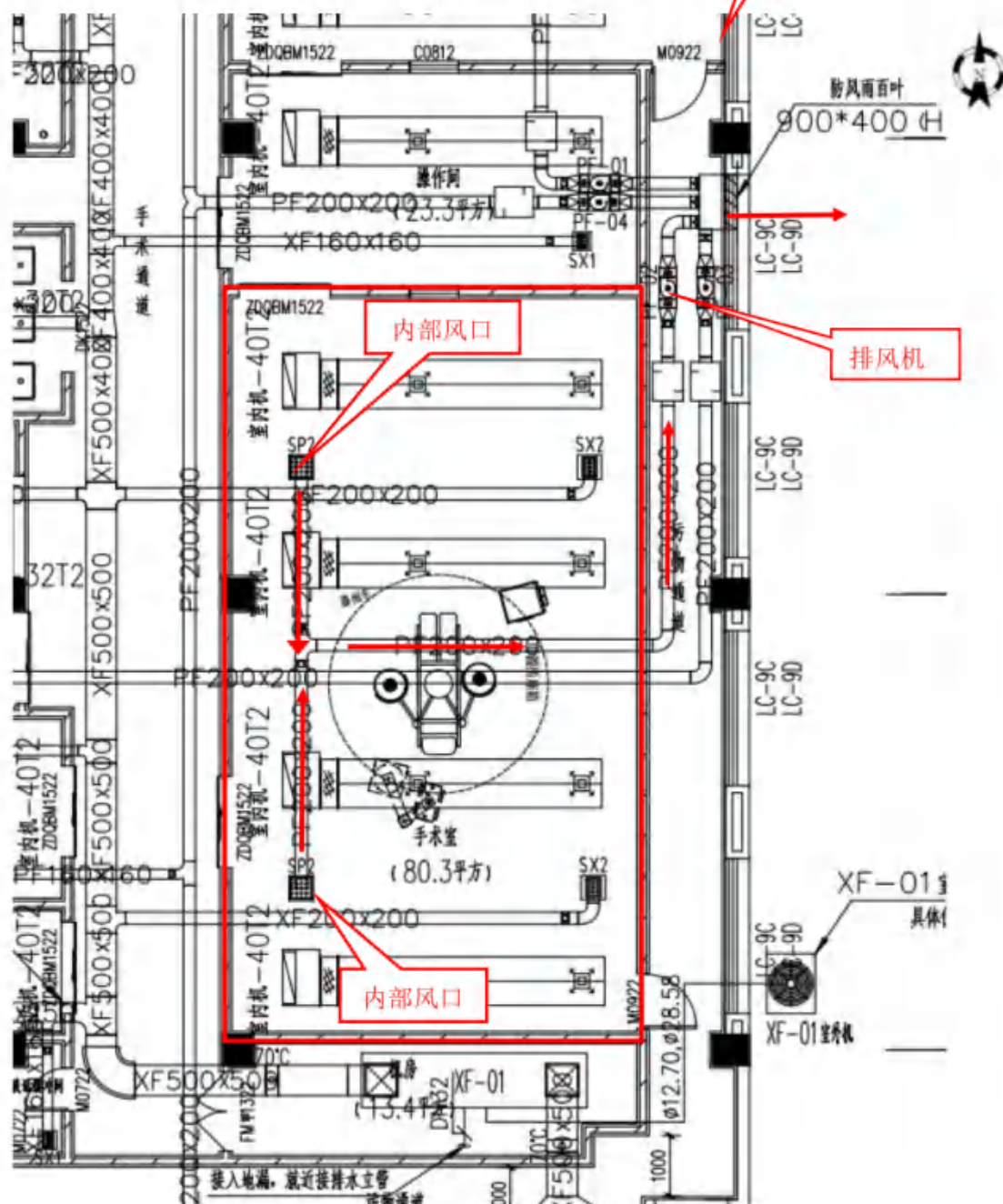
图 10-2 机房排风图
