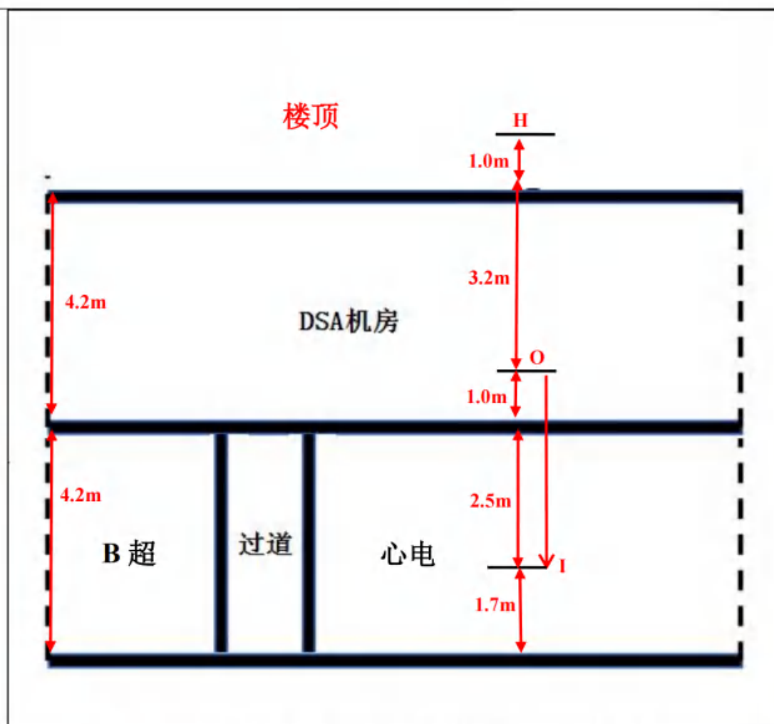
图 11-3 DSA 手术室楼上及楼下关注点示意图（剖面图）
